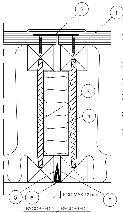
DETALJ A -1:4
