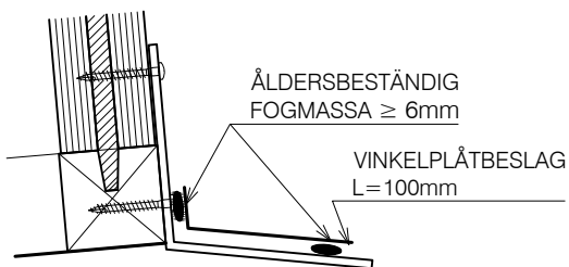
TÄTNING MELLAN L-STÅL VY FRÅN SIDAN:
