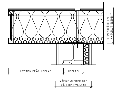
DETALJ 5 SKALA 1 : 20
