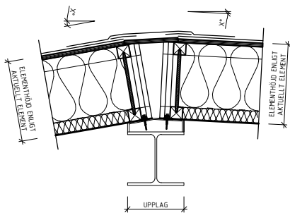
DETALJ 3 SKALA 1 : 20
