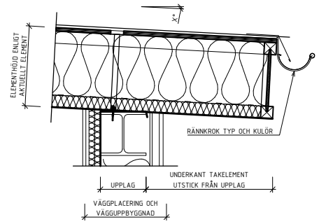
DETALJ 2 SKALA 1 : 20
