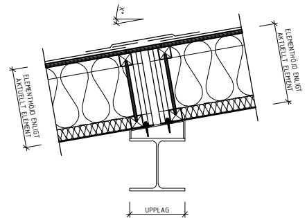
DETALJ 4 SKALA 1 : 20
