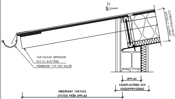
DETALJ 1 SKALA 1 : 20
