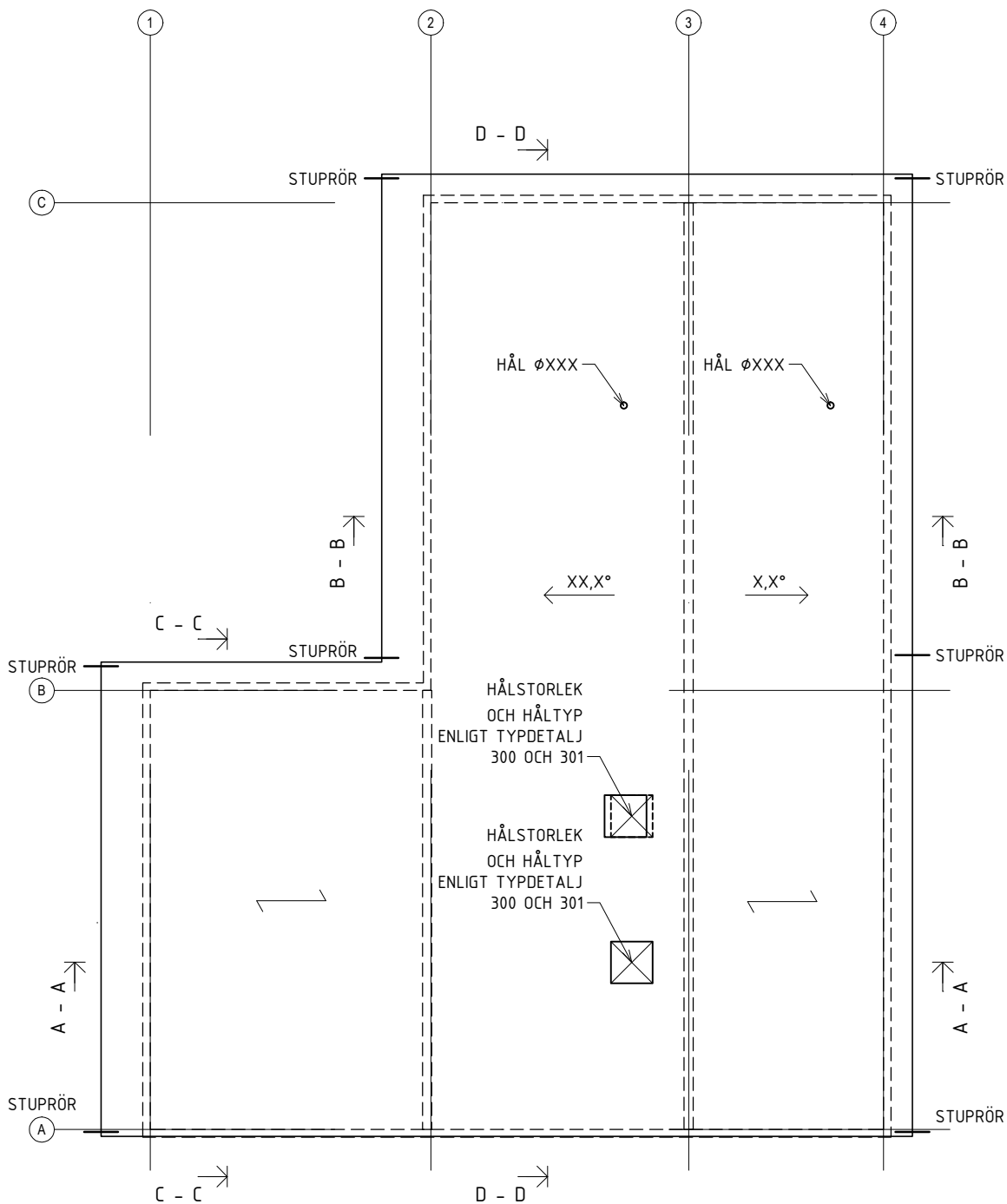
TAKPLAN SKALA 1 : 150
