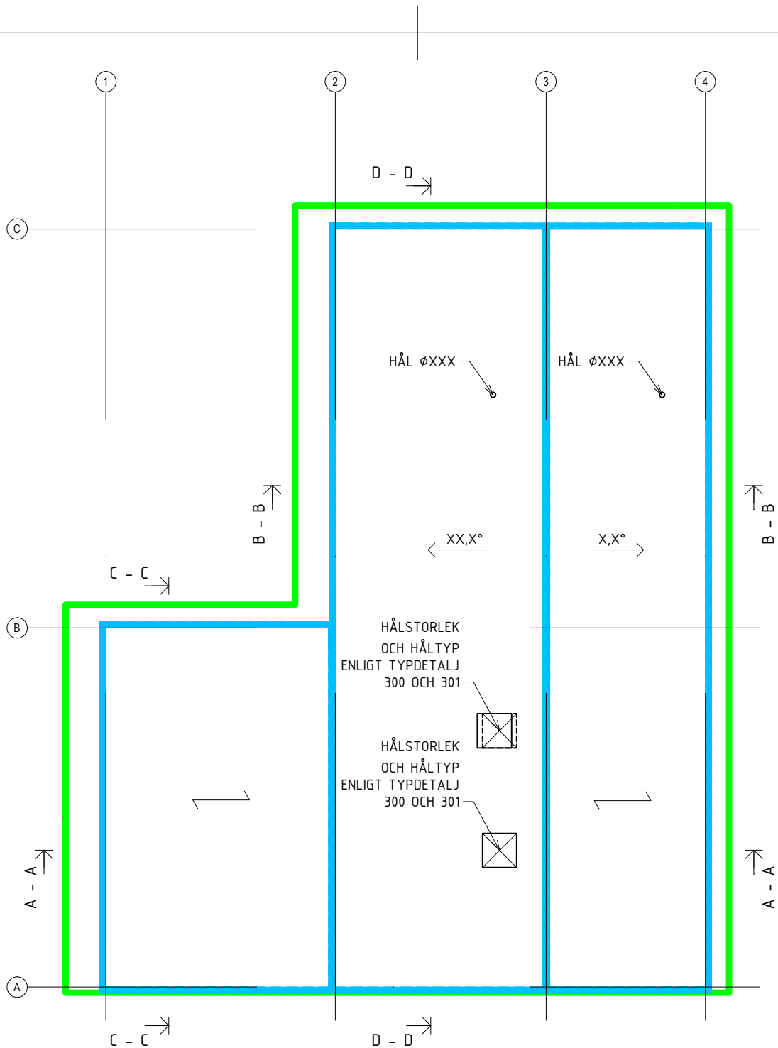
TAKPLAN SKALA 1 : 150
