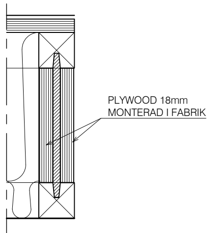
D: LIVFYLLED ELEMENTÄNDE PÅ TVÅ SIDOR
