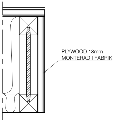
E: PLYWOODBEKLÄDD ELEMENTÄNDE
