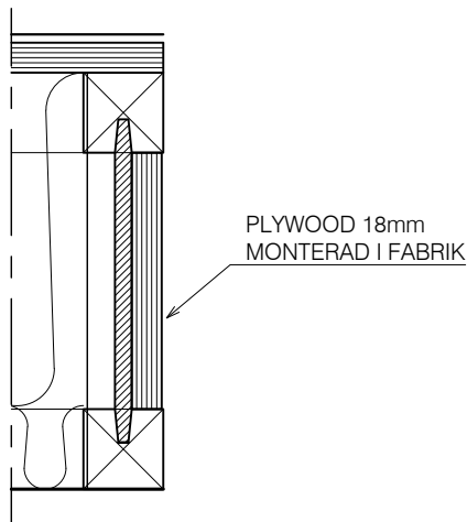
C: LIVFYLLED ELEMENTÄNDE PÅ EN SIDA
