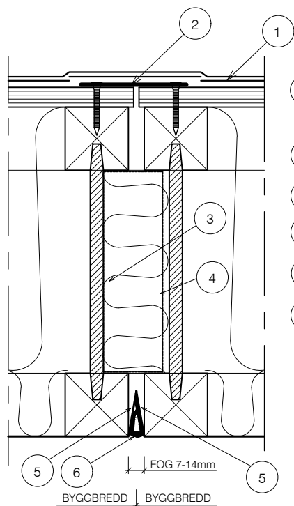
DETALJ A -1:4
