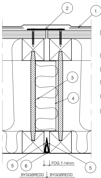
DETALJ A -1:4
